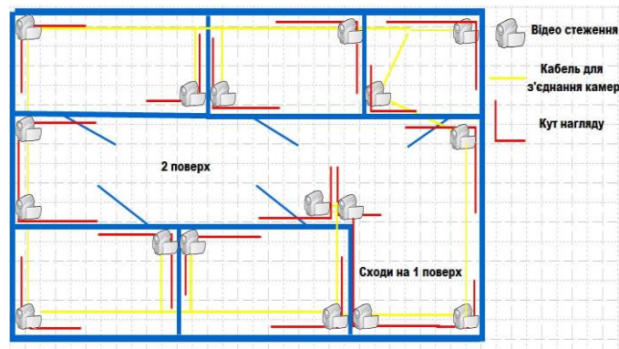
Рисунок 10 – Система відео нагляду другого поверху
