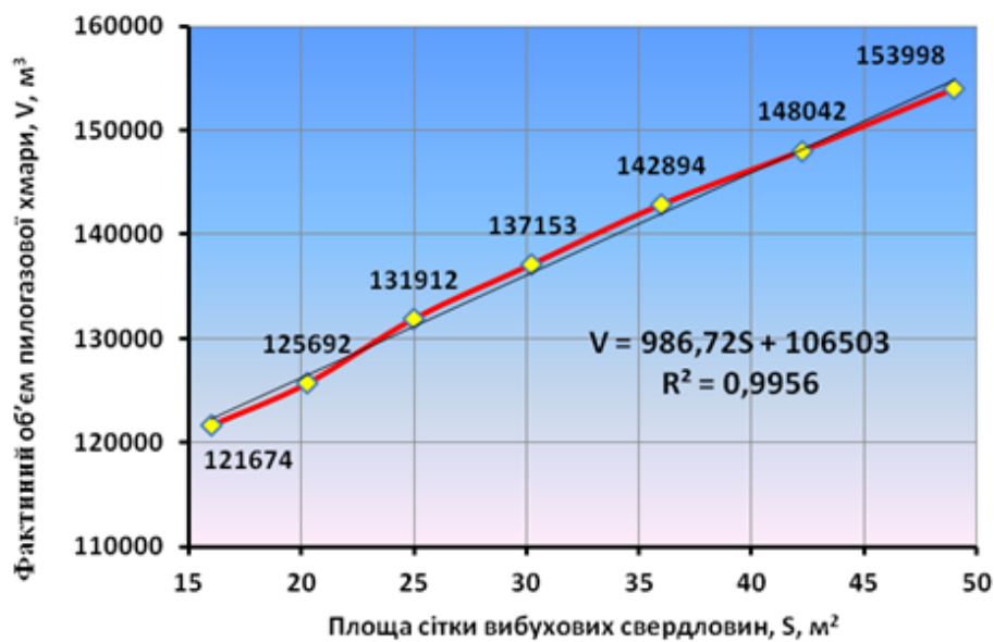
Рис. 2. Залежність фактичного об'єму пилогазової хмари від площі сітки вибухових свердловин при відбійці залізистих кварцитів
