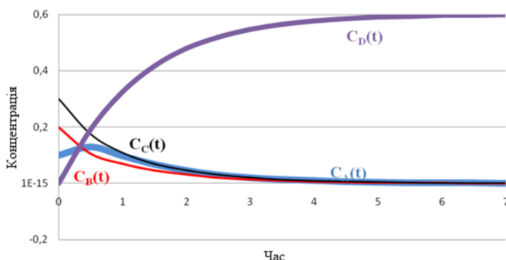
Рис. 1. Кінетичні криві залежності концентрації від часу для речовин А, В, С, D при послідовній реакції першого порядку
