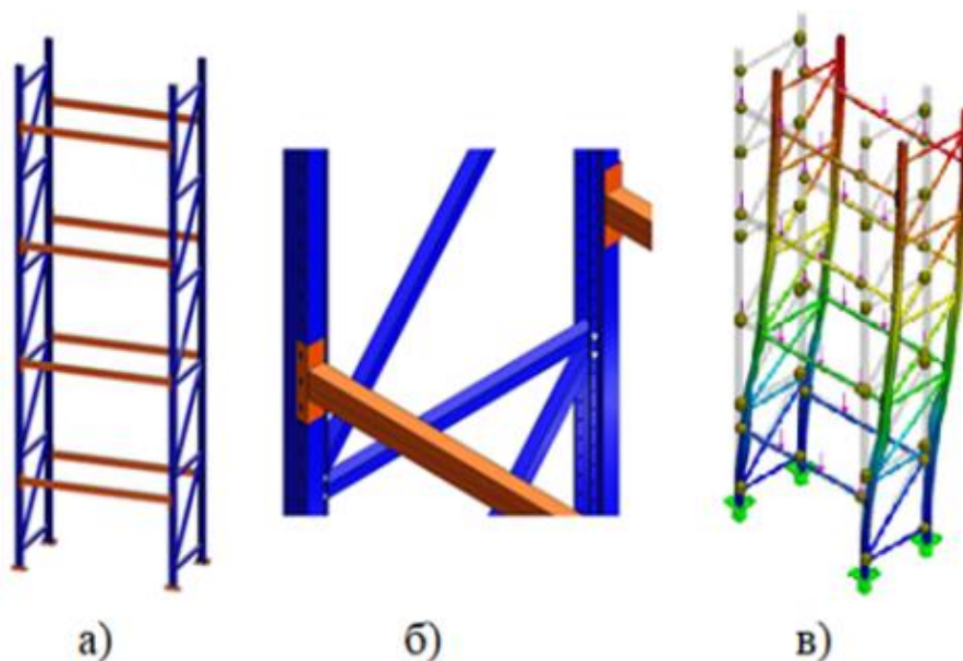
Рис. 1 - Комбінована розрахункова схема секції стелажу а) геометрична модель б) моделювання роз'ємних з'єднань в) розрахункова схема
