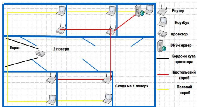
Рисунок 9 – Схема СКС мережі та пристроїв другого поверху
