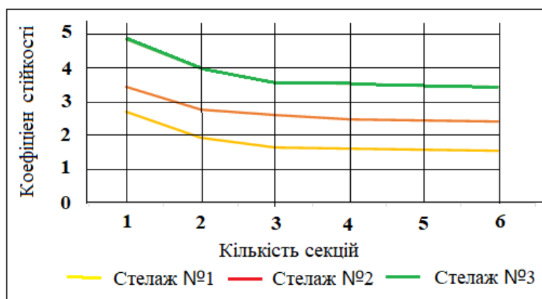
Рис. 2 - Залежність коефіцієнта стійкості від кількості секцій стелажу
