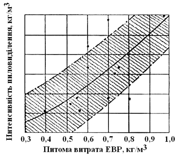
Рис. 1. Залежність інтенсивності утворення пилу від питомих витрат емульсійної ВР. Пунктирними кривими обмежена зона, в межах якої входить більша частина вихідних показників
