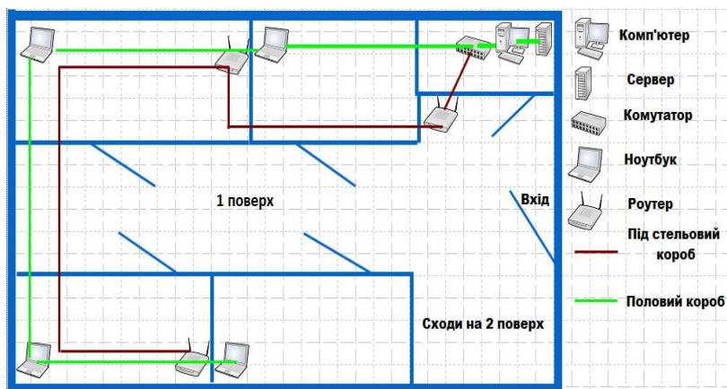
Рисунок 6 – Схема СКС мережі та пристроїв першого поверху
