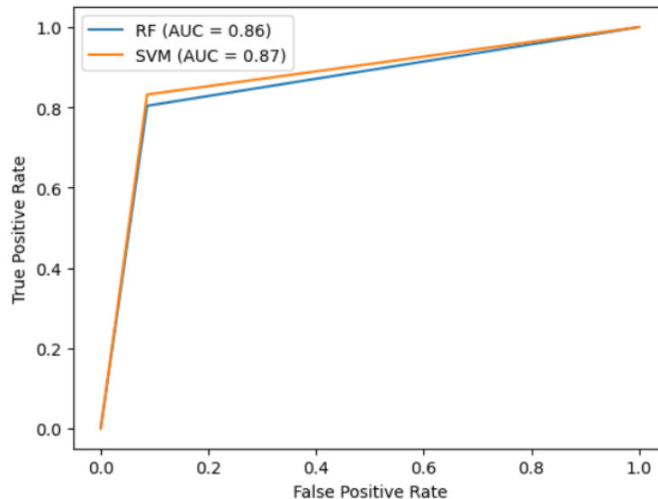
Рис. 6. Порівняння ROC кривих для моделей RF та SVM
