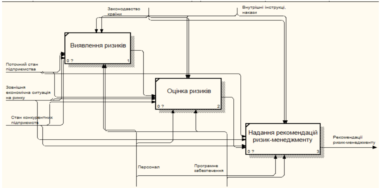
Рис. 1. IDEF0 – діаграма аналізу ризиків підприємства
