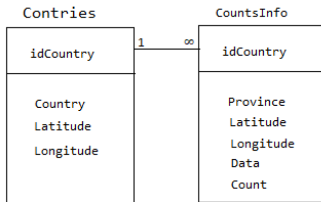
Рис. 1. Модель даних
