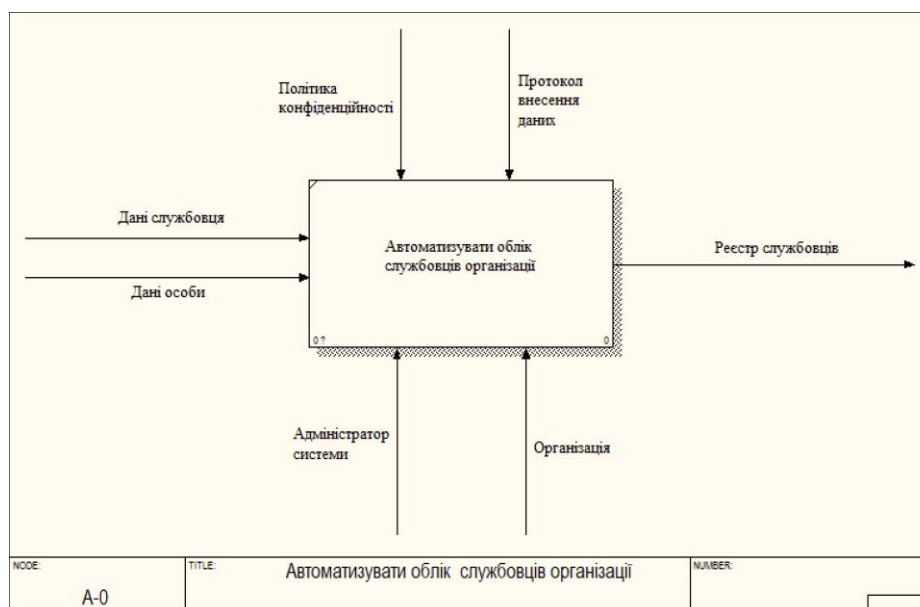
Рис. 1.1 Контекстна діаграма системи
