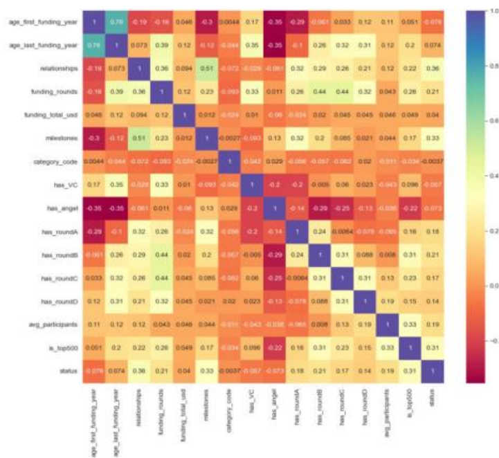
Рис. 5. Матриця кореляції
