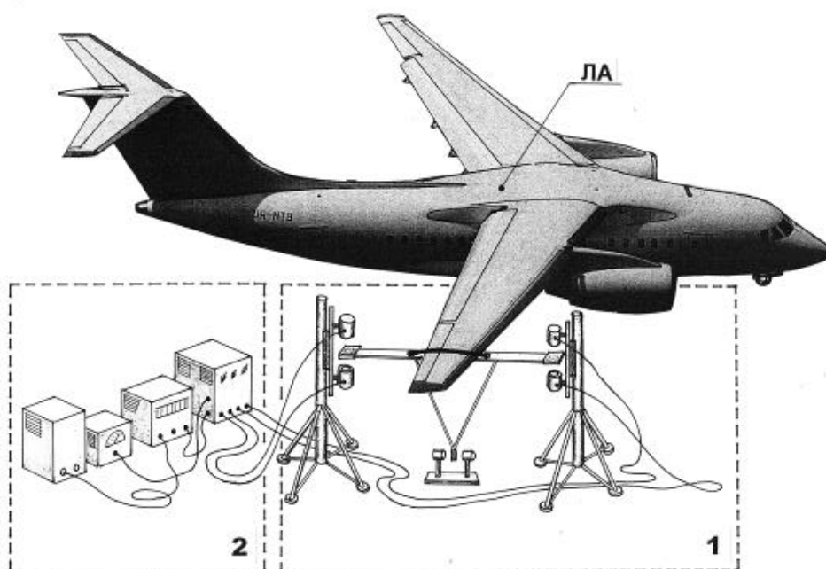
Рис. 2. Апаратура для збудження вигинних і крутних коливань крила з власною (авторезонансною) частотою.
