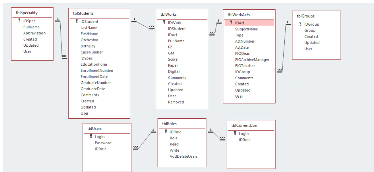
Рис. 1 Схема бази даних архіву студентських робіт
